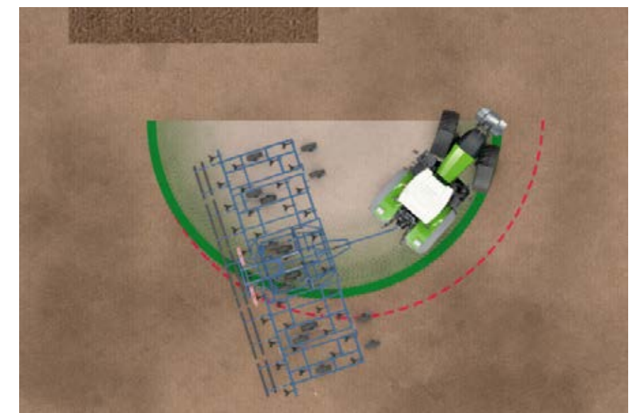
Menor radio de giro gracias al efecto "pull-in turn", por ejemplo, 6,1 m en el Fendt 930 Vario con neumáticos de serie.
