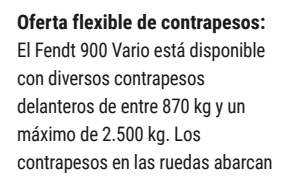
Oferta flexible de contrapesos: El Fendt 900 Vario está disponible con diversos contrapesos delanteros de entre 870 kg y un máximo de 2.500 kg. Los contrapesos en las ruedas abarcan desde 2 x 300 kg hasta 2 x 1.000 kg (2 x 1.250 kg con cultivo en hileras).
