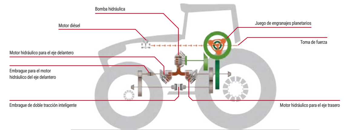
Diagrama que muestra el diseño del VarioDrive de Fendt.
